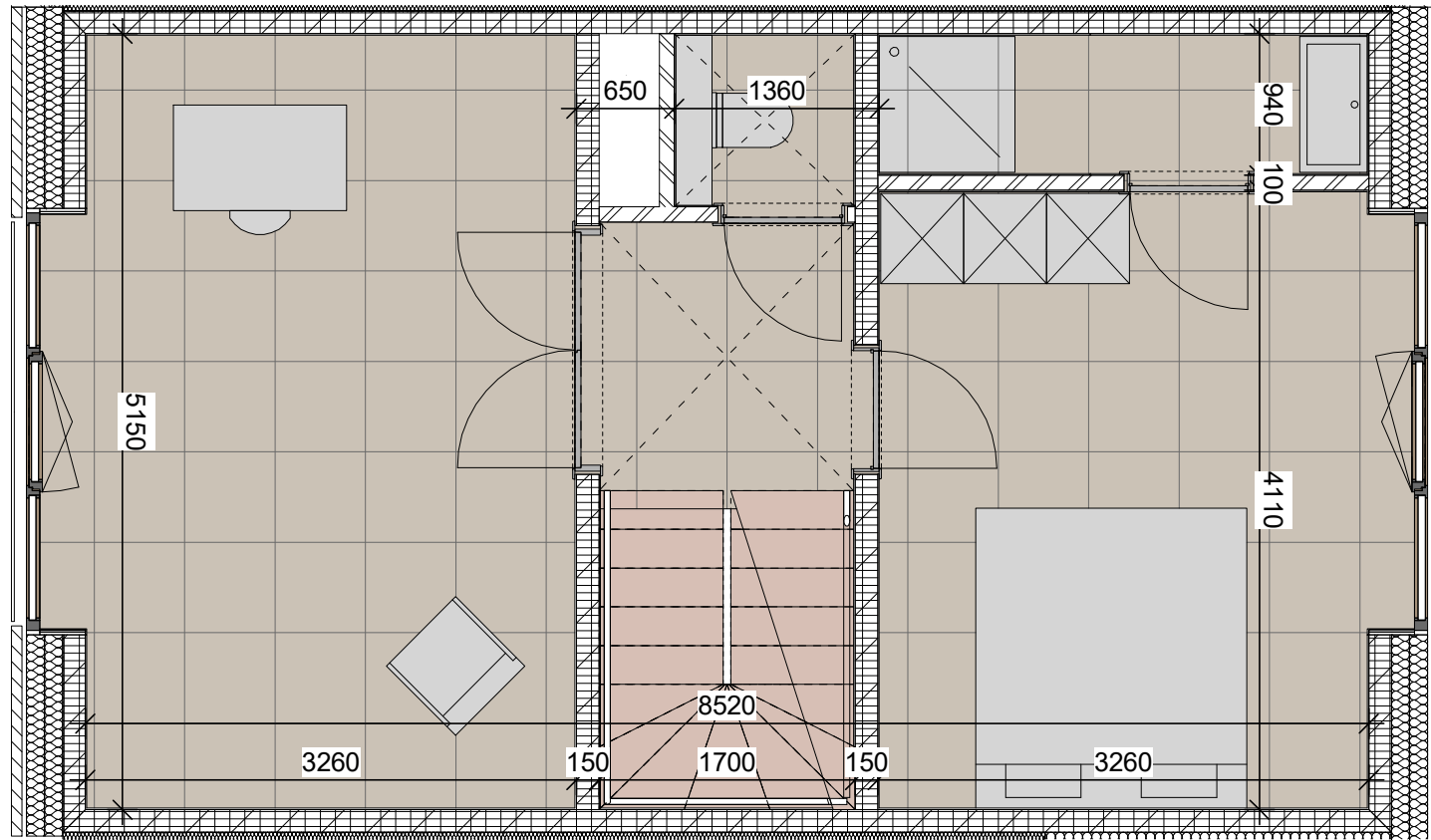
1ste verdieping
